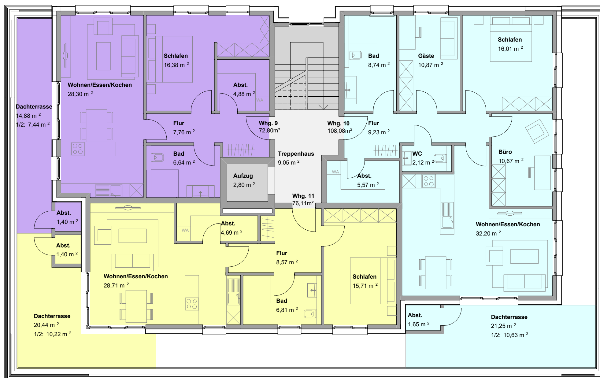
Haus 3, 2.OG
