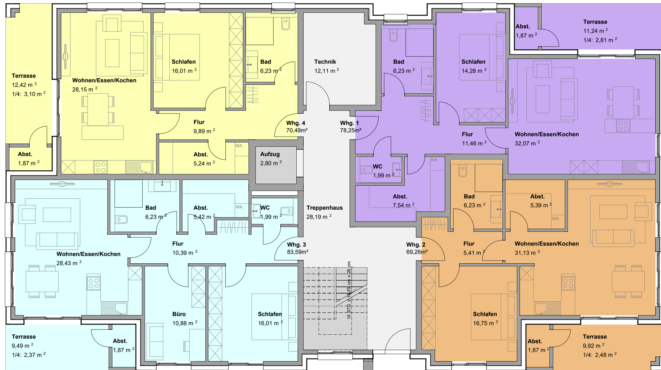
Haus 5, EG
