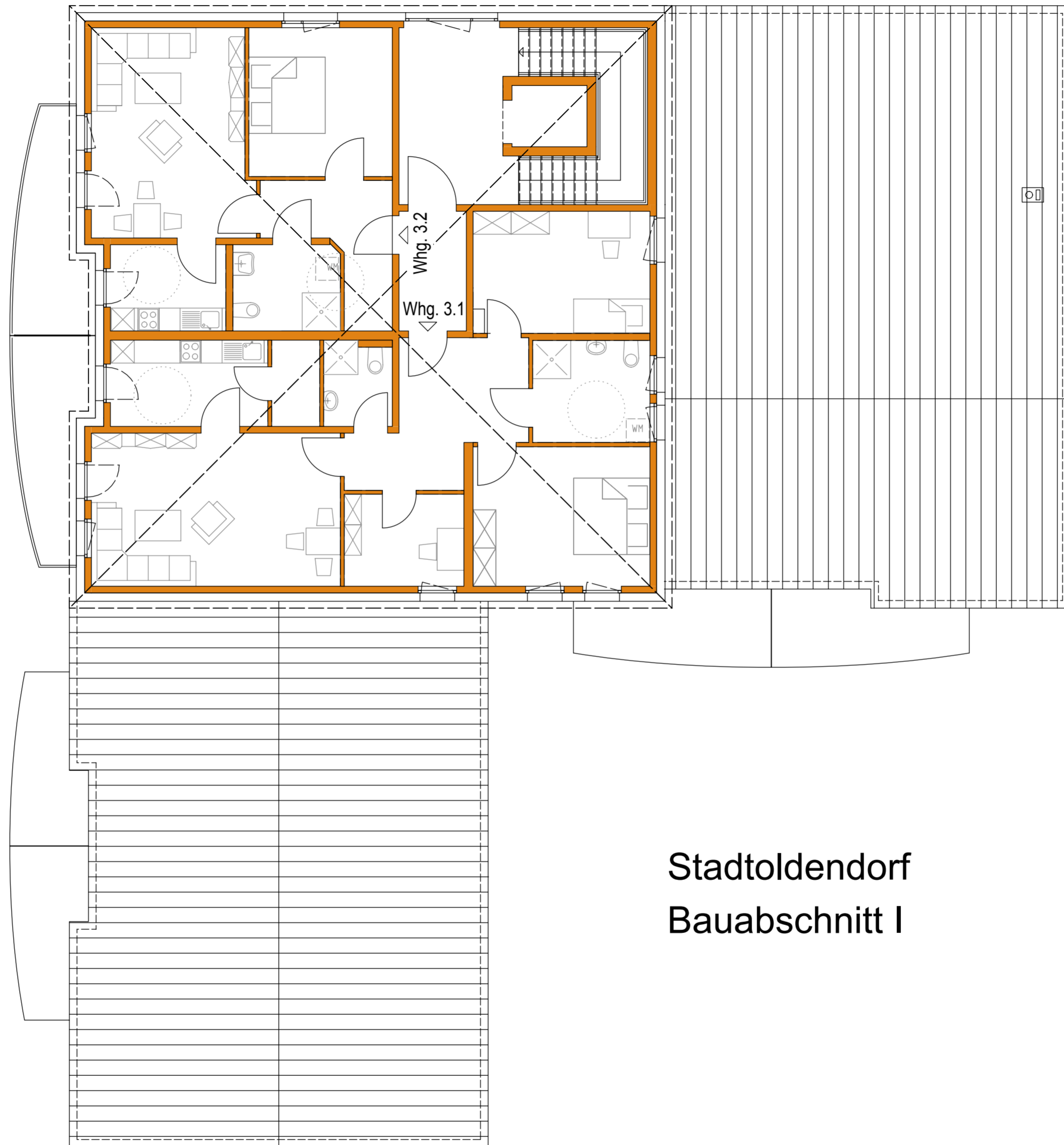
3. Obergeschoss
